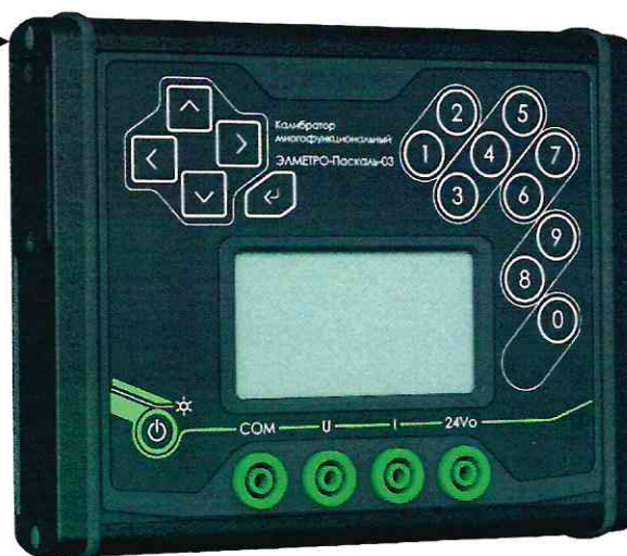
Рисунок 1 – Общий вид калибраторов и место пломбирования от несанкционированного доступа
